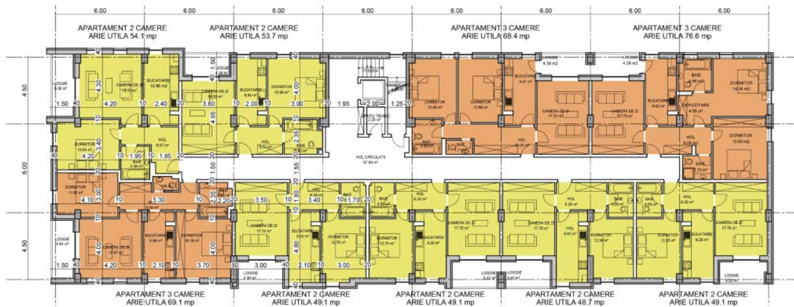
PLAN ETAJ 1-4, CORP A
